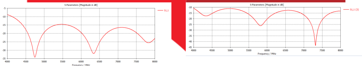
(a) (b) Gambar 3.3 Returnloss dengan Software (a) 1 Substrat, (b) 2 Substrat.
