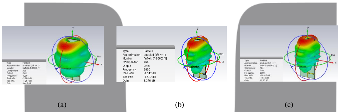
Gambar 3.4 Gain dengan Software (a) 4 Ghz, (b) 6 Ghz, (c) 8 Ghz.
