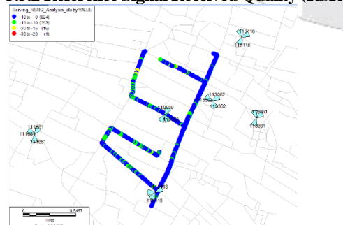
Gambar 3.4 Persebaran RSRQ Jaringan Eksisting
