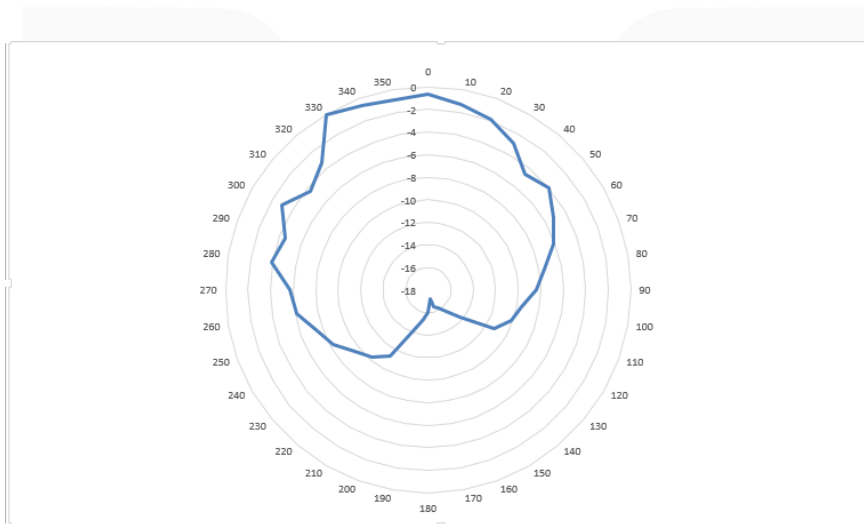
Gambar 4.5 Hasil pengukuran polarisasi
