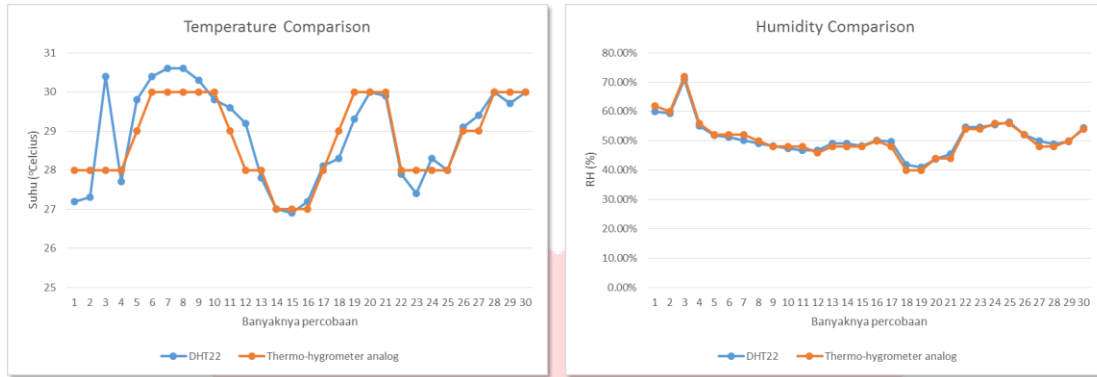
Gambar 5 Hasil Pengujian Pengukuran Suhu dan Kelembapan
