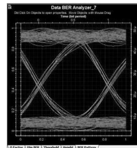
Gambar 4 Eye Diagram GPON link downstream pada titik terjauh
