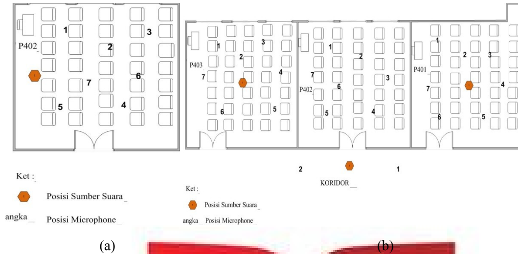
Gambar 2 Denah titik pengukuran (a) medan suara (b) insulasi suara
