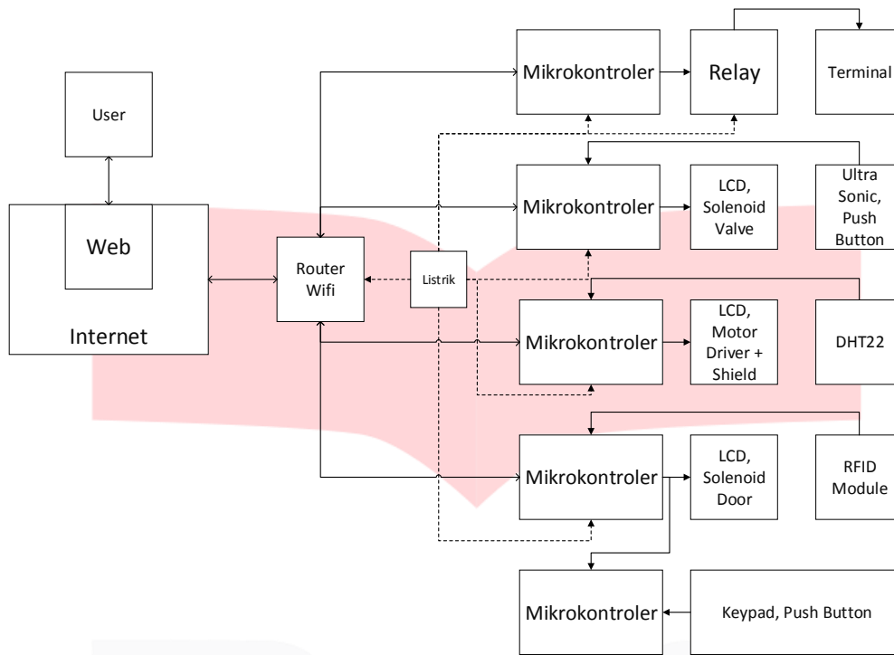
Gambar 10: Skema Perangkat
