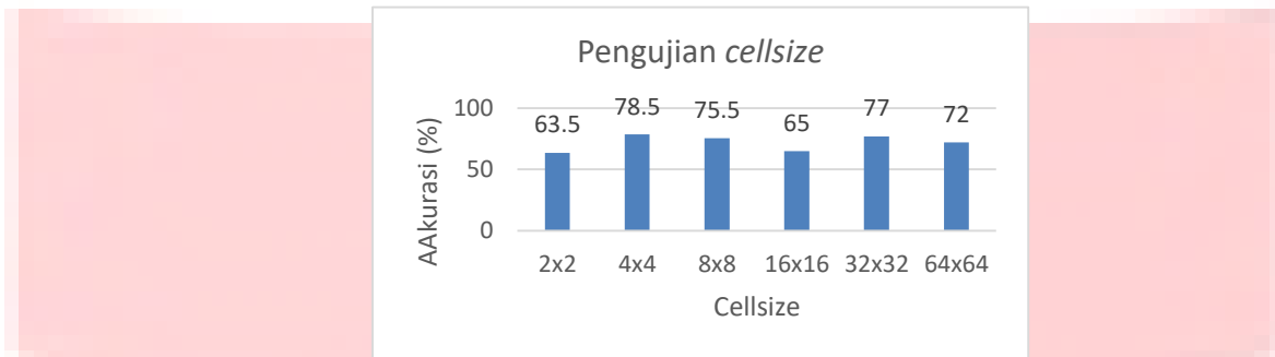
Gambar 6. Grafik hasil pengujian akurasi cell size
