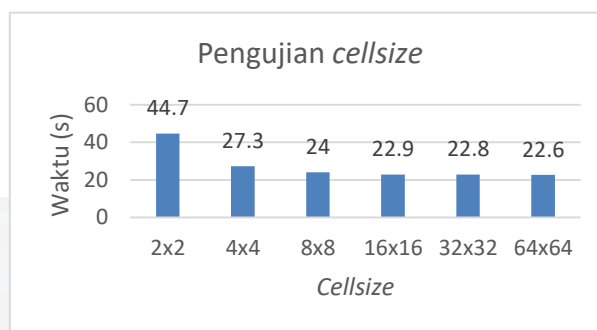
Gambar 7. Grafik hasil pengujian waktu cell size
