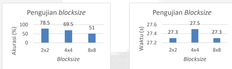
Gambar 8. Grafik hasil pengujian akurasi dan waktu block size
