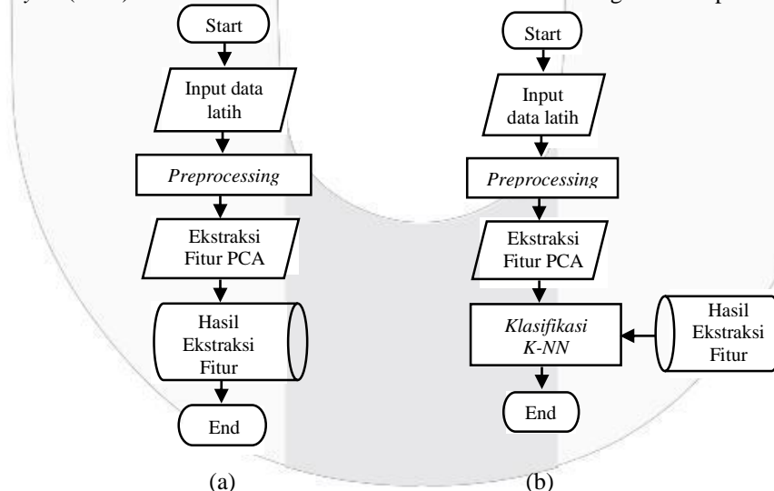
Gambar 3.2 Diagram alir perancangan sistem klasifikasi colon cancer (a) Data Latih (b) Data Uji
