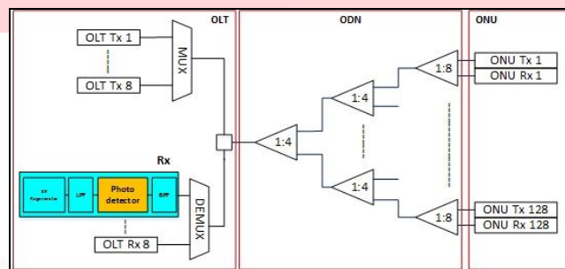
Gambar 4. Arsitektur Skenario 128 ONU
