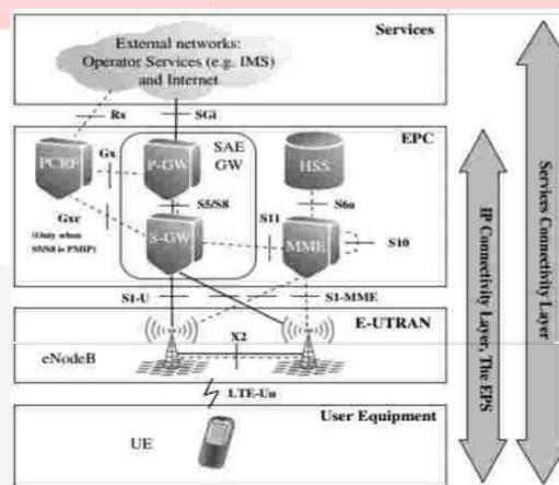
Gambar 1 Arsitektur LTE
