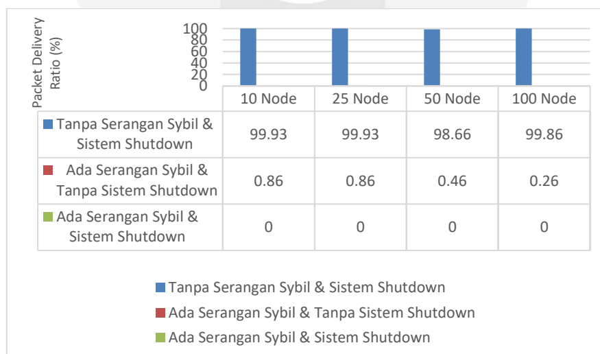
Grafik 1 Packet Delivery Ratio dengan hasil pada setiap skenario
