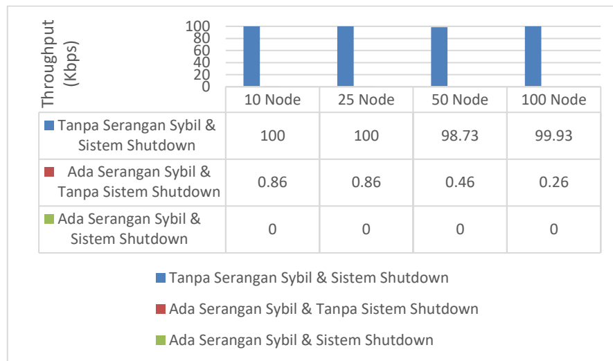
Grafik 2 Throughput dengan hasil pada setiap skenario
