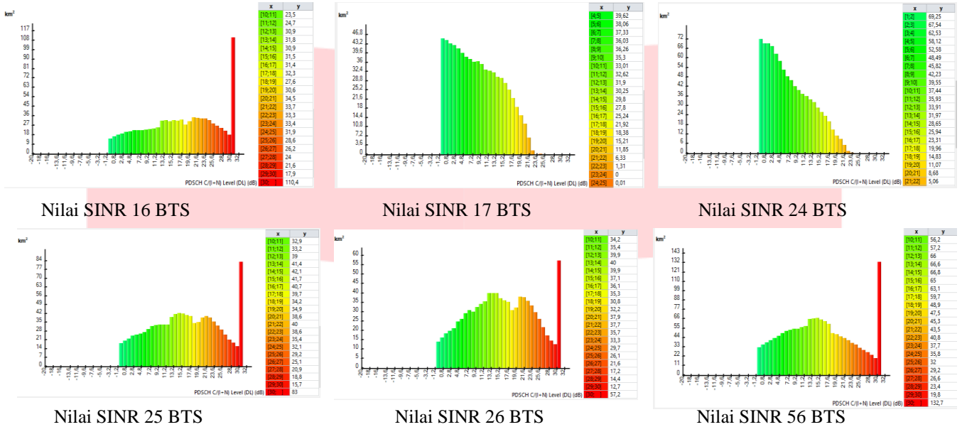
Gambar 4.5 Nilai SINR dengan Bandwidth 5Mhz
