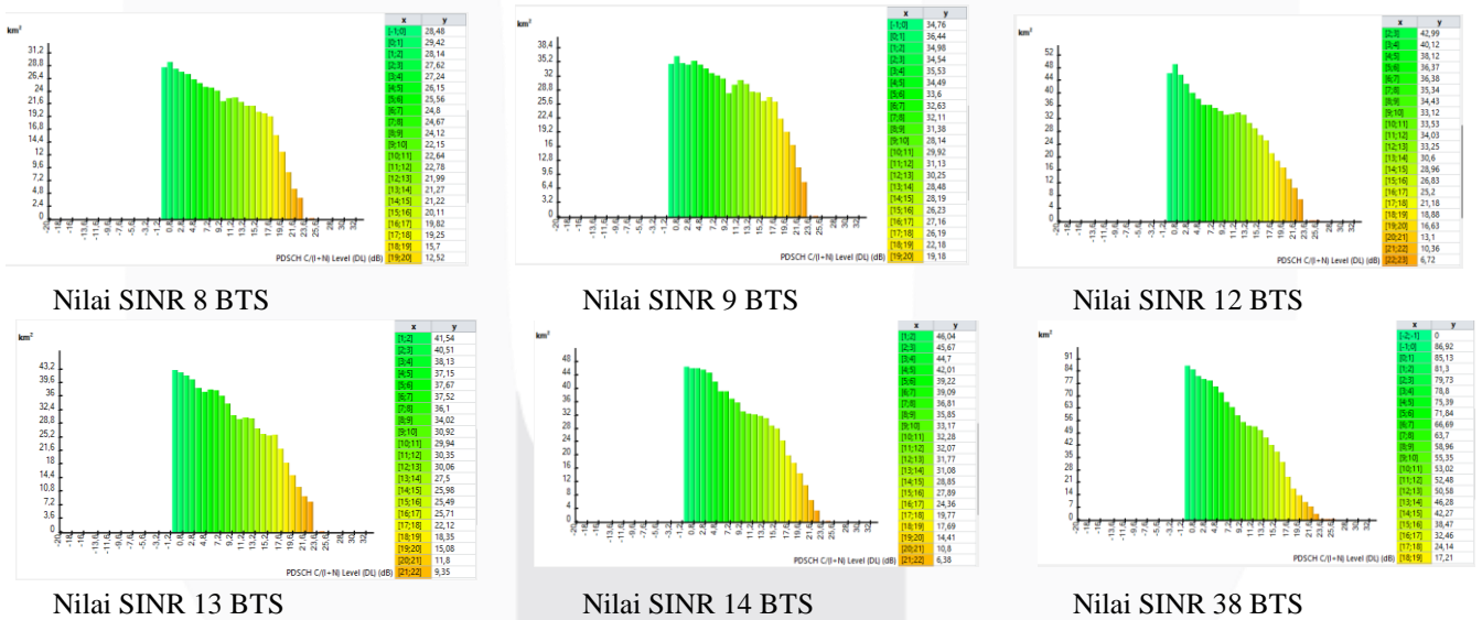
Gambar 4.5 Nilai SINR dengan Bandwidth 10Mhz
