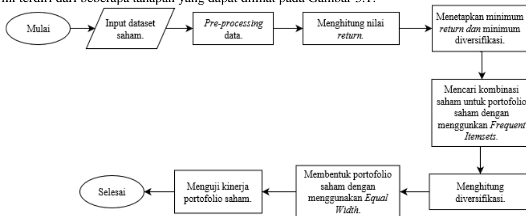
Gambar 3.1 Flowchart pemilihan portofolio saham.
