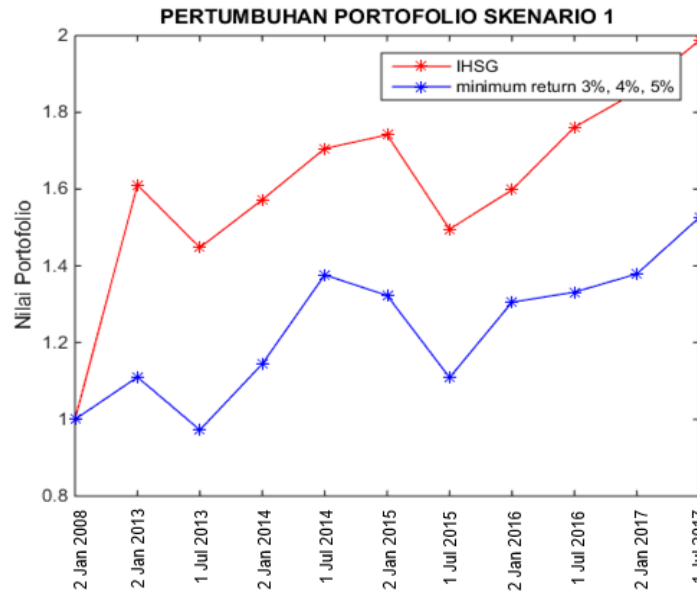
Gambar 4.1 Grafik pertumbuhan portofolio skenario 1 dengan minimum return 3%.
