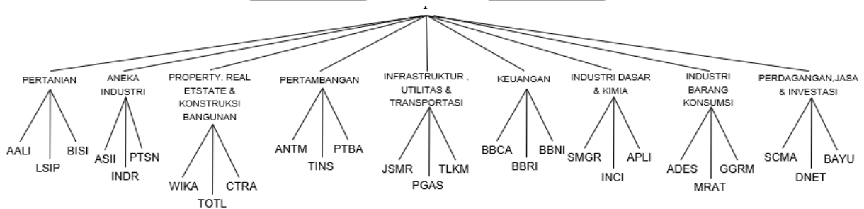
Gambar 2.1 Pengelompokan data saham pada sektor pasar.
