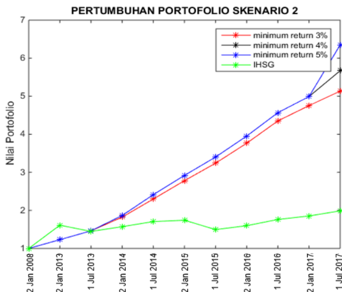
Gambar 4.2 Grafik pertumbuhan portofolio skenario 2 dengan minimum return 3%.
