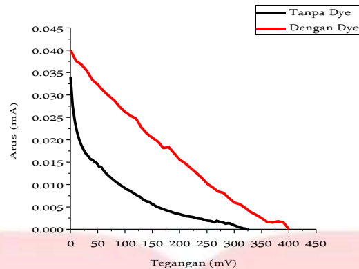
Gambar 3.3 Perbandingan kurva I-V sel surya \text{TiO}_2 dengan dan tanpa perendaman dye.
