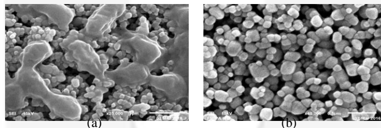
Gambar 3.4 Hasil uji SEM, (a) sampel \text{TiO}_2 dye buah naga perbesaran 25.000x, (b) sampel \text{TiO}_2 tanpa dye perbesaran 40.000x.
