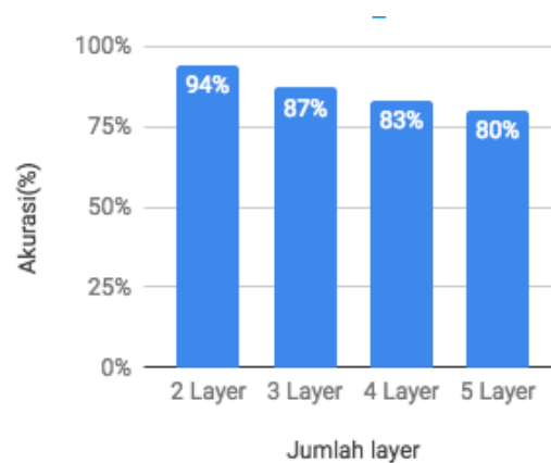
Gambar 8. Hasil Pengujian Pengaruh Jumlah Layer SDAE
