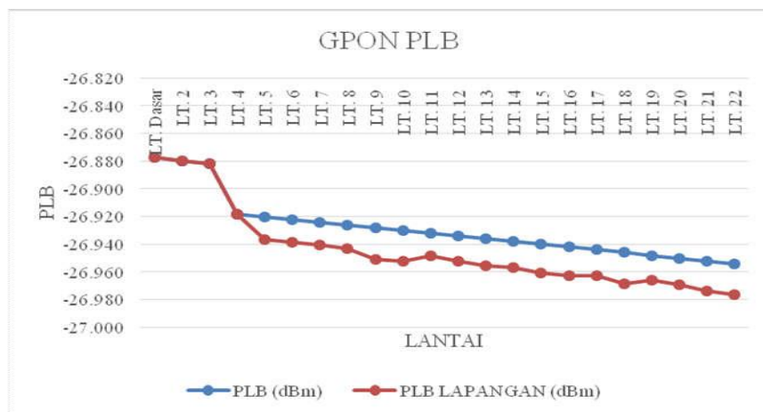
Gambar 3. 4 Hasil Perbandingan Simulasi GPON dan Data Lapangan
