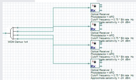
Gambar 9 Blok penerima
