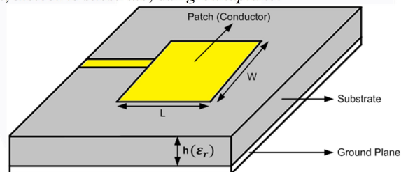
Gambar 2.1 Antena Mikrostrip
