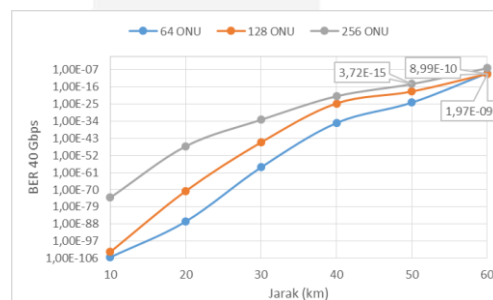
Gambar 16 BER 40 Gbps Upstream Penguat
