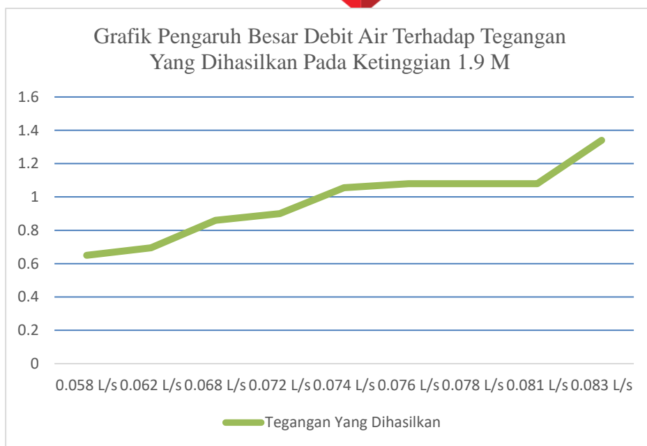
Grafik 3.1 Grafik Tegangan Terhadap Debit Air Ketinggian 1.9M
