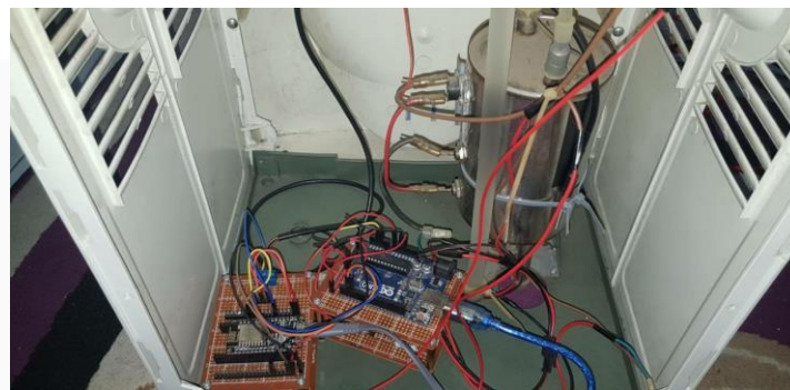
Gambar 3-2 Hardware Keseluruhan dari Dispenser.
