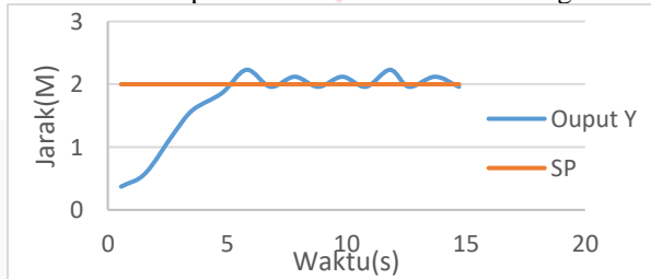
Grafik 3.6 Respons Kontrol Pada Sumbu Y dengan PID
