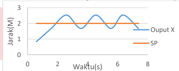
Grafik 3.5 Respons kontrol Pada Sumbu x Dengan PID
