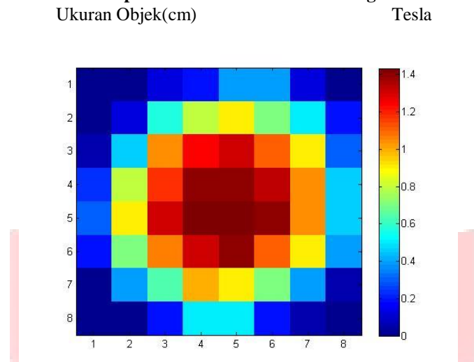
Gambar 4. 1 Distribusi medan magnet koil segienam 8x8 Berdasarkan hasil eksperimen yang sudah diolah menjadi image , kehomogenan distribusi medan magnet dengan bentuk koil segienam sebesar 0.61161.
