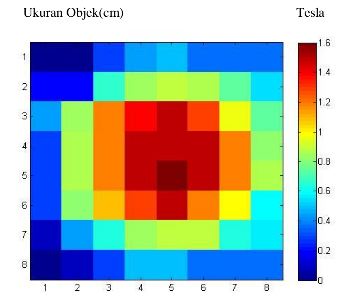
Gambar 4. 2 Distribusi medan magnet koil persegi 8x8 Berdasarkan hasil eksperimen yang sudah diolah menjadi image , kehomogenan distribusi medan magnet dengan bentuk koil persegi sebesar 0.66458.
