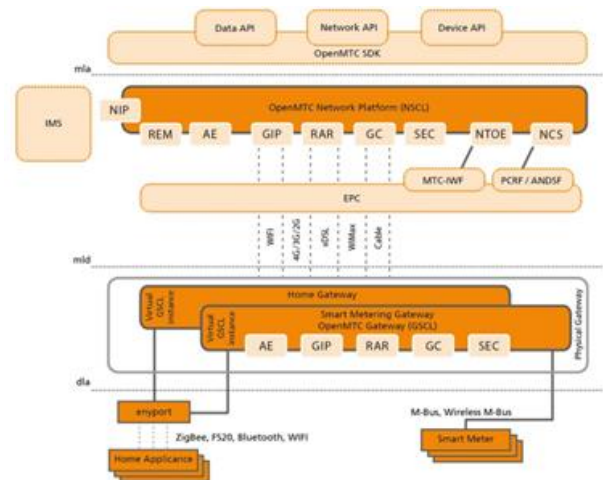
Gambar 1. Arsitektur OpenMTC
