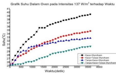
Gambar 3.5 Grafik suhu dalam oven pada intensitas 137 W/m 2 terhadap waktu
