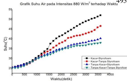
Gambar 3.4 Grafik suhu air pada intensitas 880 W/m 2 terhadap waktu
