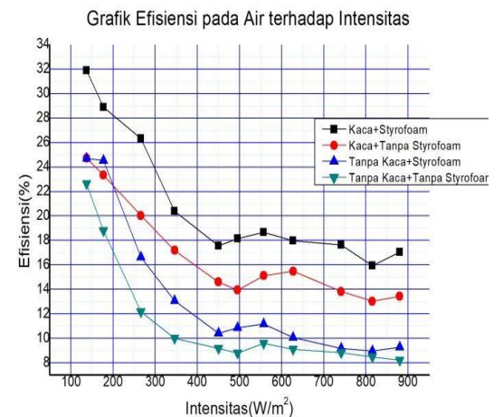
Gambar 3.10 Grafik efisiensi pada air
