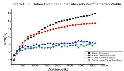
Gambar 3.6 Grafik suhu dalam oven pada intensitas 495 W/m 2 terhadap waktu
