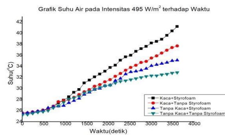
Gambar 3.3 Grafik suhu air pada intensitas 495 W/m 2 terhadap waktu
