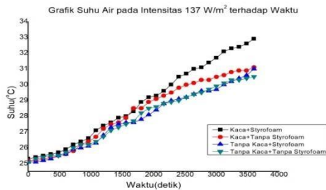
Gambar 3.2 Grafik suhu air pada intensitas 137 W/m 2 terhadap waktu
