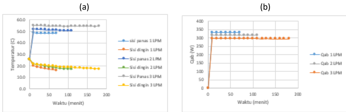
Gambar 3.3 (a) Temperatur sisi panas dan dingin TEC (b) nilai penyerapan kalor oleh sisi dingin TEC ( \dot{Q}_{ab} )
