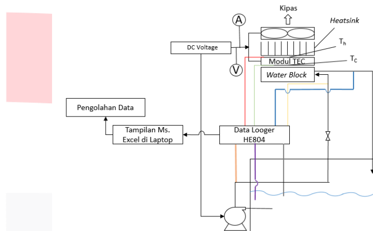
Gambar 2.3 Skema pengukuran penelitian
