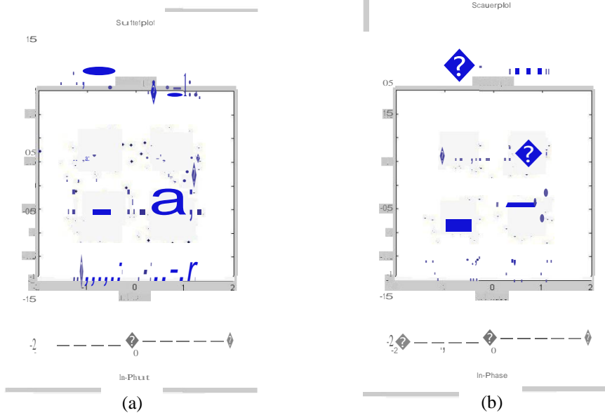
Gambar 6. Diagram konstelasi MISO-OFDM kondisi user dengan kecepatan 50km/jam, (a) tanpa SIC dan (b) dengan SIC
