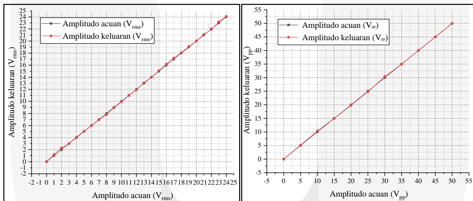
Gambar grafik keluaran amplitudo gelombang kotak
