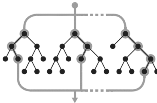
Gambar 4. Ensembled pohon-pohon yang digunakan dalam Random Forest
