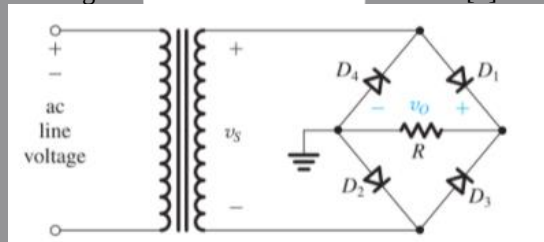
Gambar 2. Rangkaian Penyearah[8]
