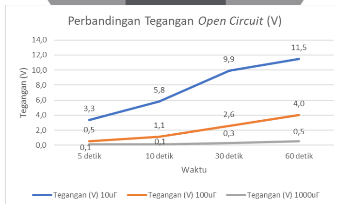
Gambar 10. Grafik Perbandingan Tegangan Open Circuit pada Kapasitor 10 \mu\text{F} , 100 \mu\text{F} , dan 1000 \mu\text{F}
