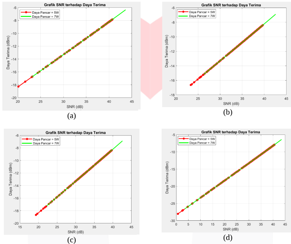
Gambar 3 Grafik daya terima terhadap SNR yang diposisikan (a) 0^\circ (b) 10^\circ (c) 15^\circ (d) 30^\circ .
