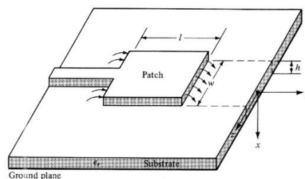
Gambar 2.1. Antena Mikrostrip
