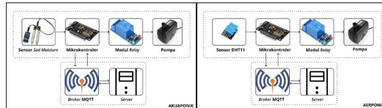
Gambar 4. Sistem Kontrol Akuaponik dan Aeroponik.
