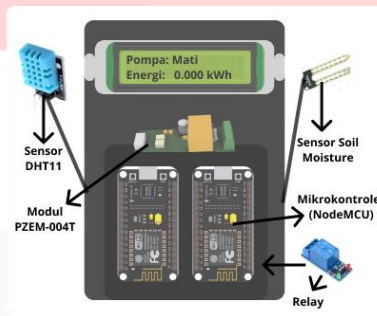
Gambar 3. Perancangan Alat.
