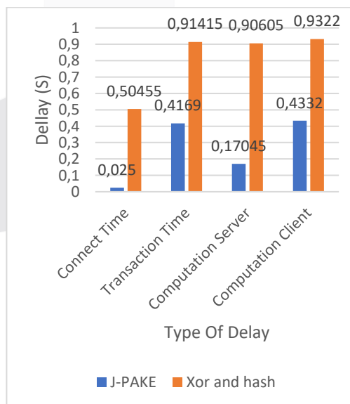
Gambar 8 Grafik rata - rata delay pada kinerja perangkat client maksimum
