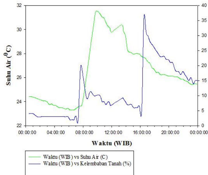
Gambar 8 Pengukuran Suhu Air dan Kelembaban Tanah Pada Tanggal 18/6/21
