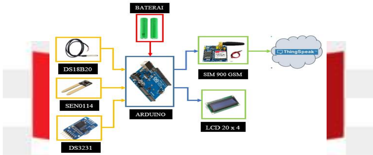
Gambar 2 Desain Perangkat Keras
