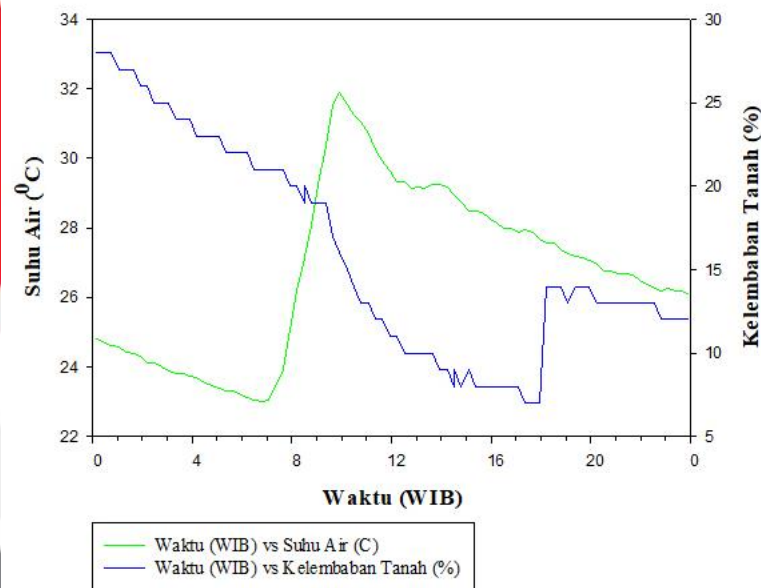
Grafik 6 Pengukuran Suhu Air dan Kelembaban Tanah Pada Tanggal 22/6/21
