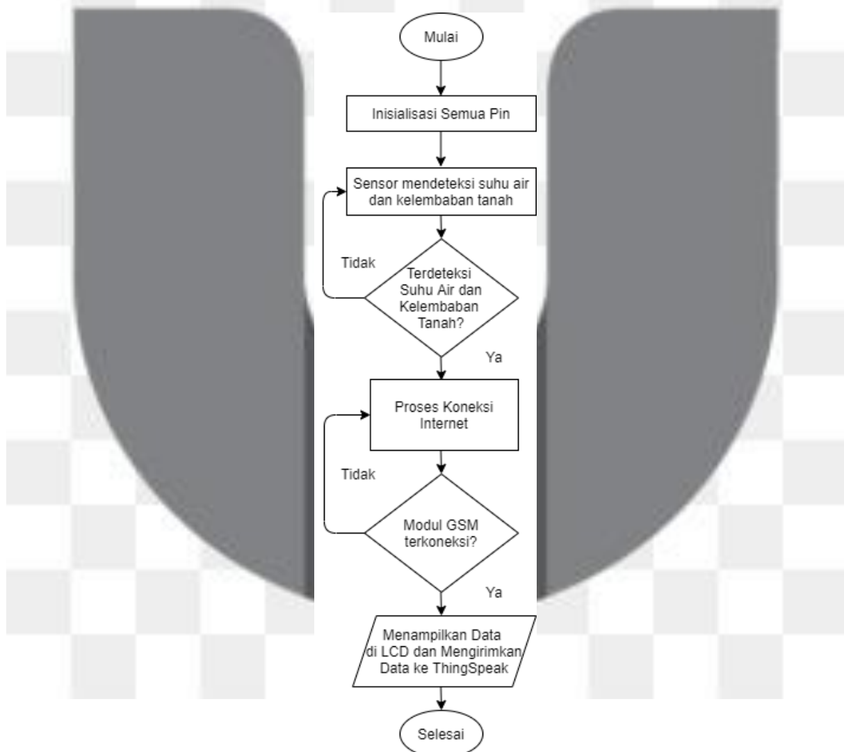
Gambar 3 Diagram Alir Sistem Pemantauan
