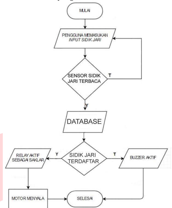
GAMBAR 3.4 FlowChart Alur Kerja Sistem
