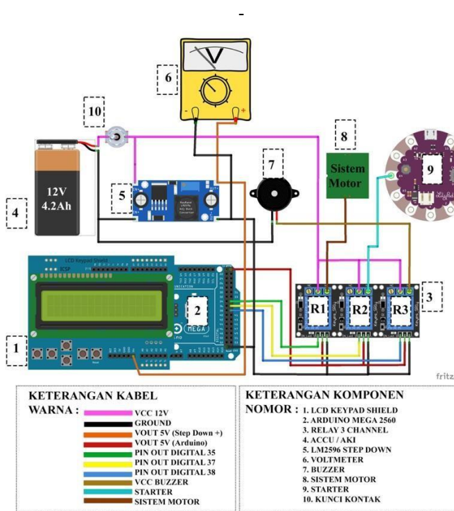
GAMBAR 3.6 Rangkaian Catu Daya Dan Relay
