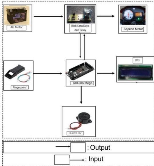
GAMBAR 3. 1 Desain Sistem
