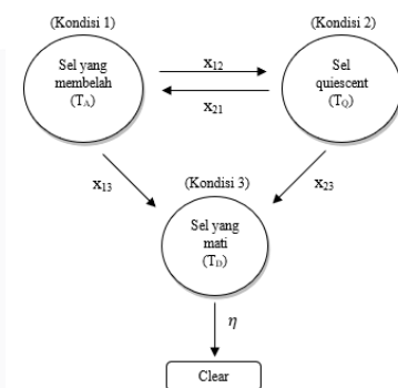
Gambar 1. Sistem interaksi tiga komponen
