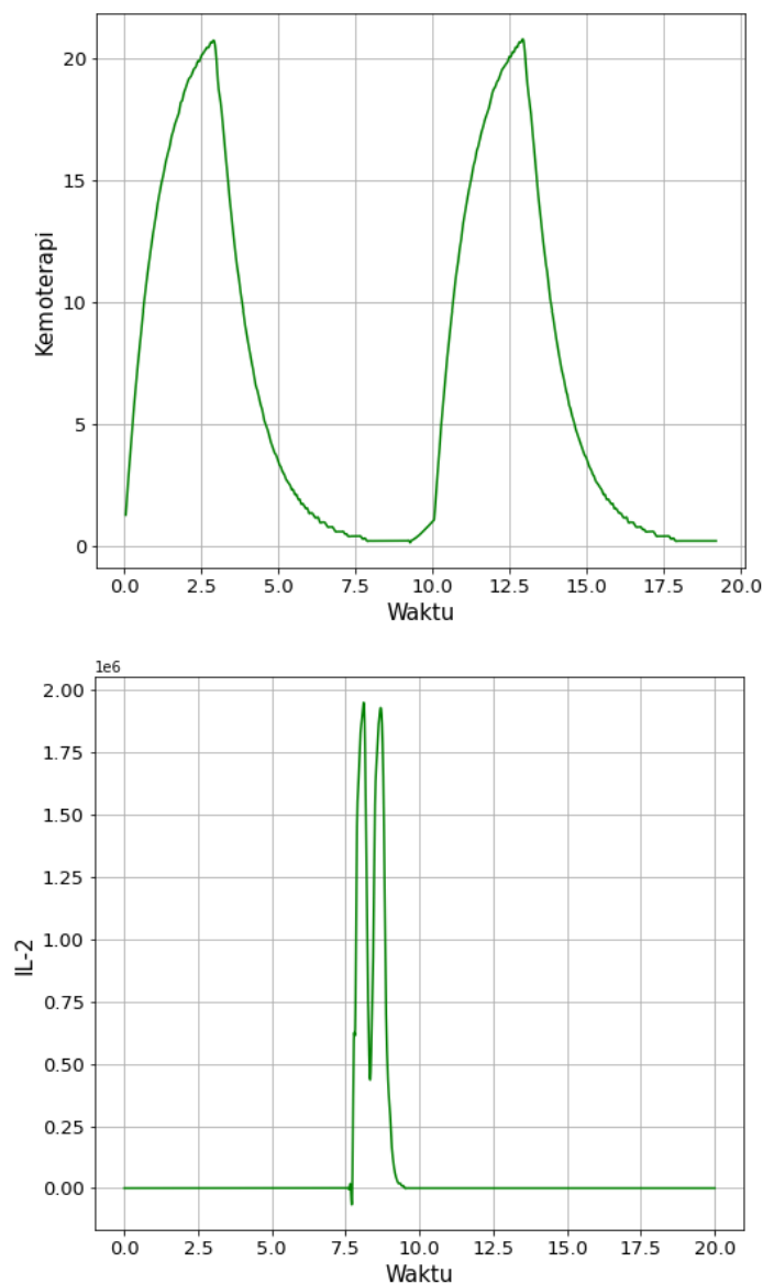
Gambar 5. Konsentrasi pengobatan kemoterapi v_m (atas) dan konsentrasi pengobatan imunoterapi v_i (bawah)
