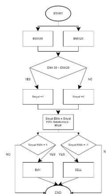
GAMBAR 3. 6 FLOWCHART PERHITUNGAN INDIKATOR EMA DAN RULES JUAL/BELI
