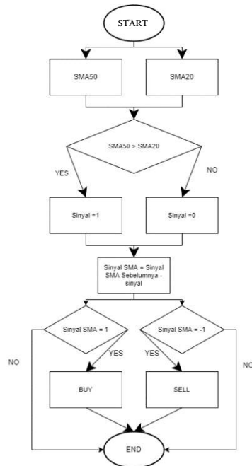
GAMBAR 3. 5 FLOWCHART PERHITUNGAN INDIKATOR SMA DAN RULES JUAL/BELI
