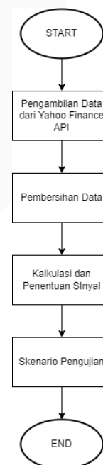
GAMBAR 3. 1 FLOWCHART GAMBARAN UMUM SISTEM PREDIKSI HARGA SAHAM
