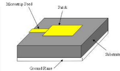
GAMBAR 2.2 (Saluran Mikrostrip Feed Line)
