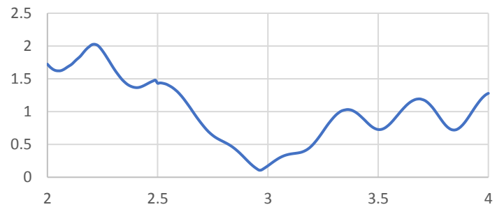
GAMBAR 4.6 (Grafik VSWR Antena Realisasi.)
