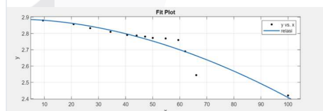
GAMBAR 4.10 (Grafik Relasi Kadar Air Dengan Pergeseran Frekuensi.)
