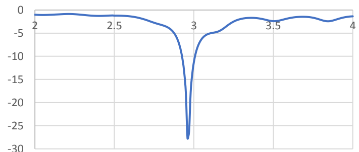
GAMBAR 4.7 (Grafik Return Loss Antena Realisasi.)
