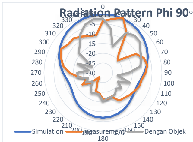
GAMBAR 4.11 (Grafik Perbandingan Pola Radiasi Elevasi.)
