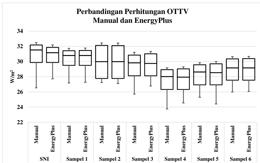
GAMBAR 3.1. (Perbandingan Perhitungan OTTV Manual dan EnergyPlus)
