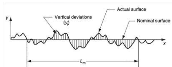
GAMBAR 1 (Deviasi dari nominal surface yang digunakan dalam dua definisi surface roughness .)
