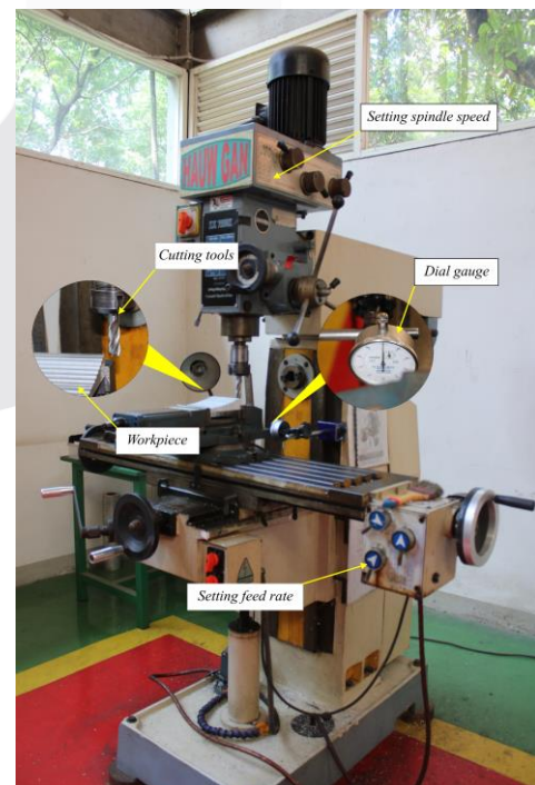
GAMBAR 3 ( Setup pemesinan)
