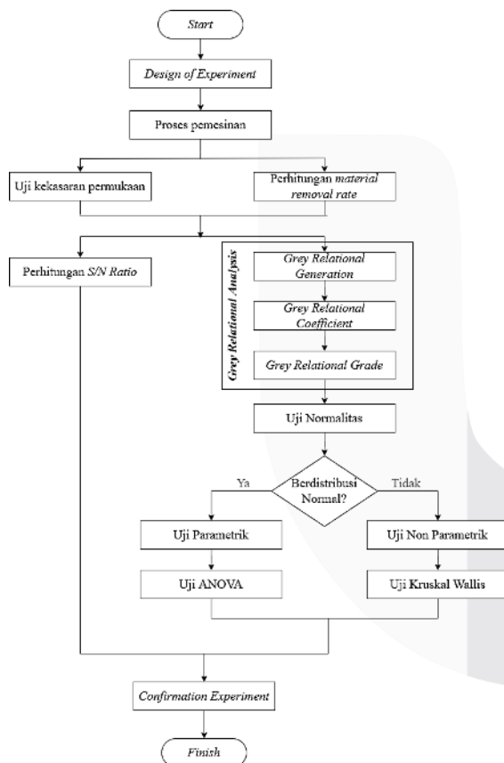
GAMBAR 2 (Metodologi penelitian)
