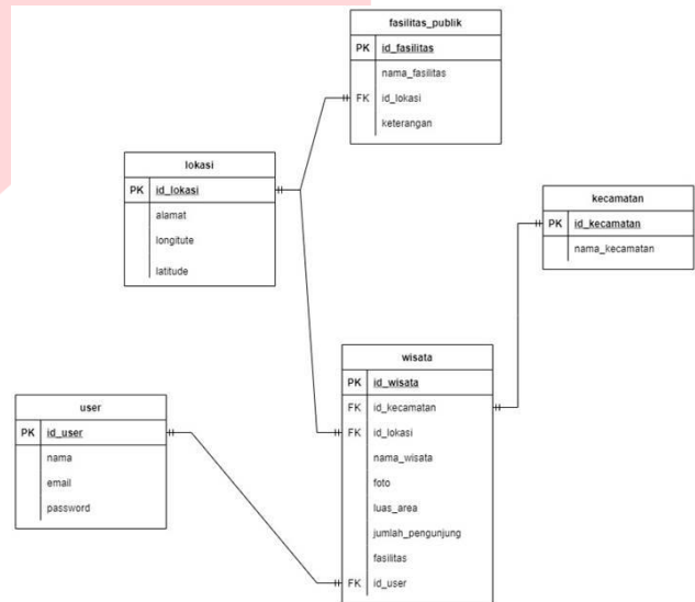
GAMBAR 7 (ERD)
