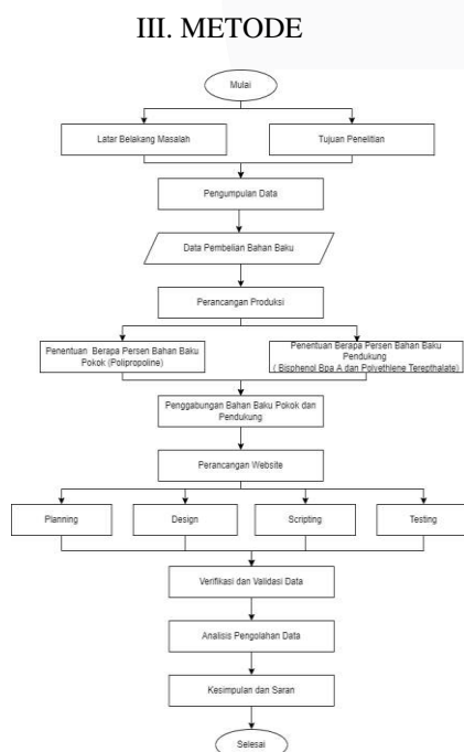
GAMBAR 1 (Sistematika Perancangan)
