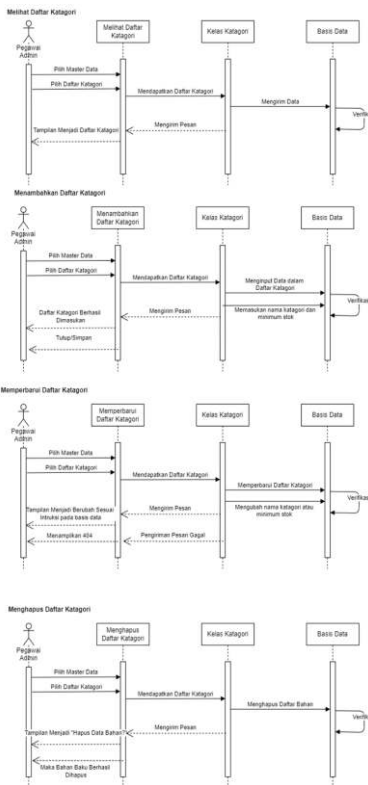
GAMBAR 26 (Diagram Sequence Daftar Kategori)
