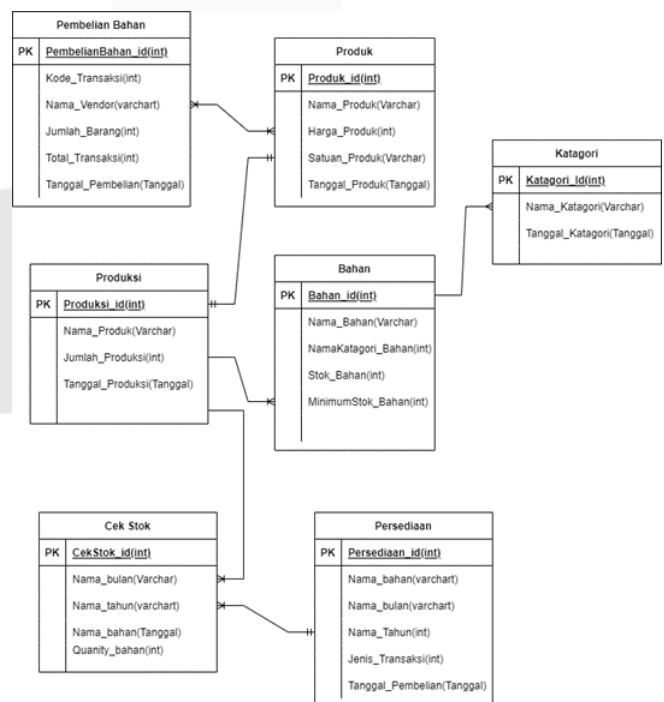
GAMBAR 2 (ERD)
