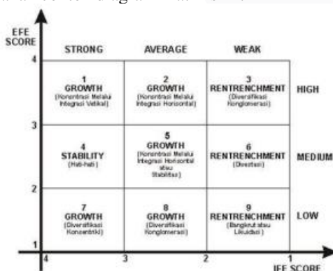
GAMBAR 1 (Matriks IE)
