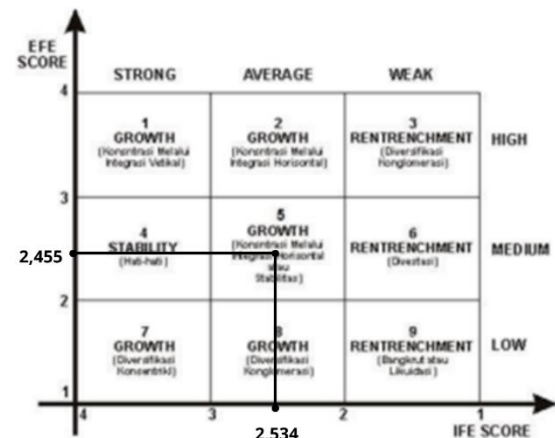
GAMBAR 4 (Matriks IE)
