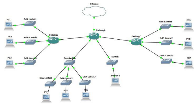
GAMBAR 6 TOPOLOGI EKSISTING
