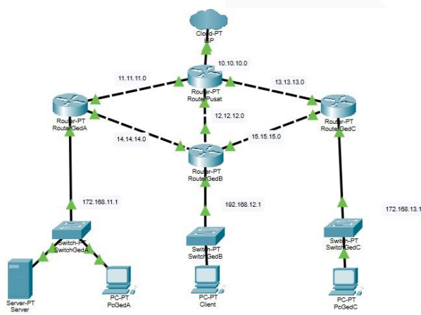
GAMBAR 9 TOPOLOGI SIMULASI
