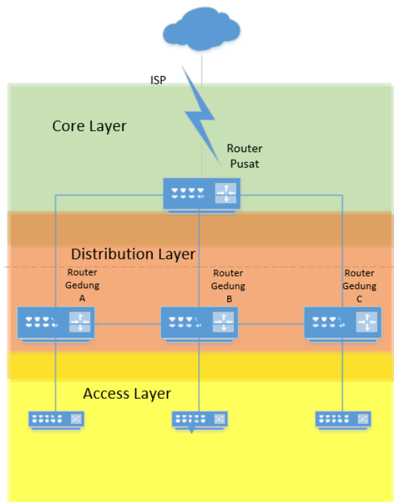
GAMBAR 8 DESAIN JARINGAN USULAN
