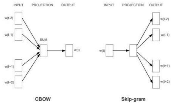
FIGURE 1 ARSITEKTUR CBOW DAN SKIP-GRAM[5]
