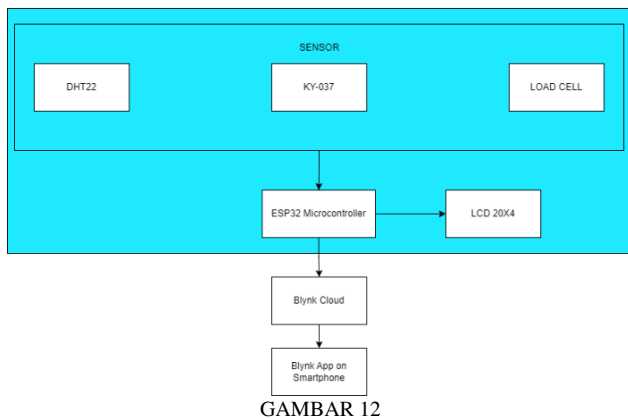
GAMBAR 12 Gambaran Umum Sistem Keseluruhan
