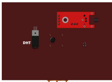
GAMBAR 18 Desain Tampak Dalam Kandang
