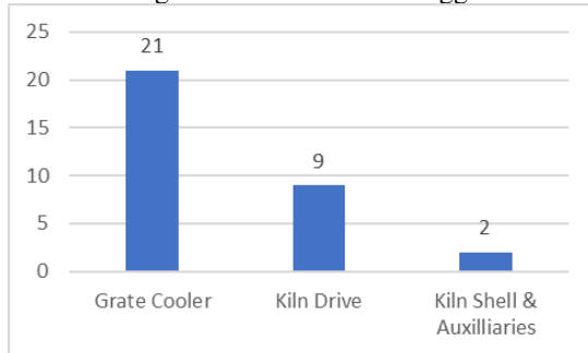
GAMBAR 2. Frekuensi kerusakan mesin pada Unit kiln
